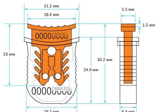
Вид спереди
