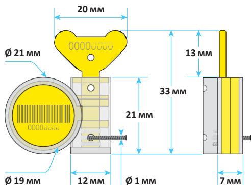
Вид спереди
