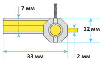
Вид снизу
